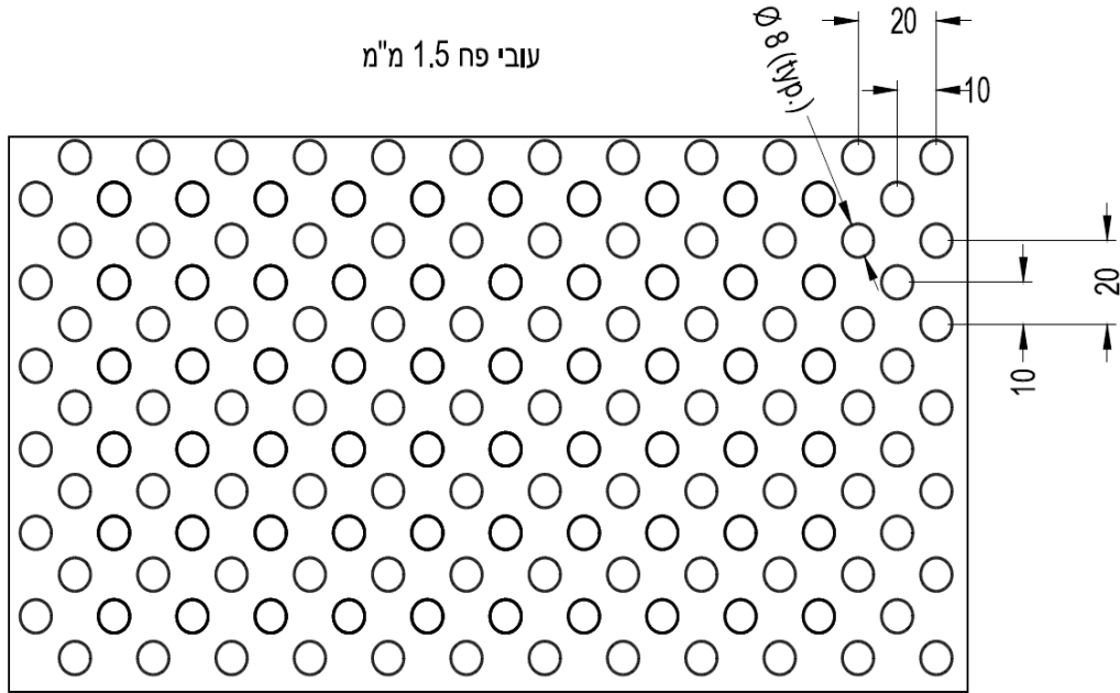
ציור מס. 1 - רשת כיסוי לתאורה ופתחי מזגו
